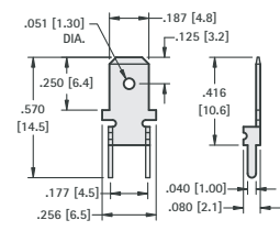
.187 (4.8) TAB
