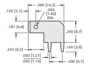
.187 (4.8) TAB
