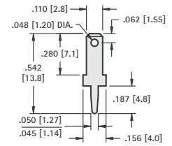
.110 (2.8) TAB
